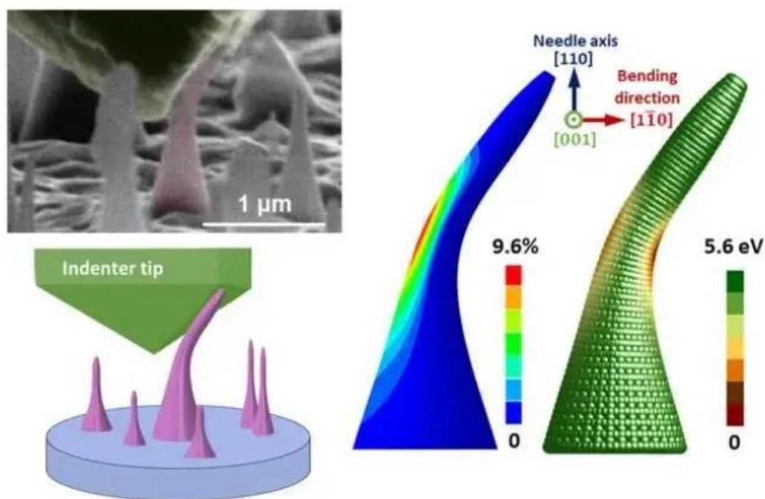
左上：纳米针被弯曲的电子显微镜图像 右图：电子显微镜下纳米针被弯曲的图像
